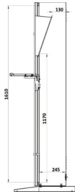
Wymiary wewnętrzne komory
