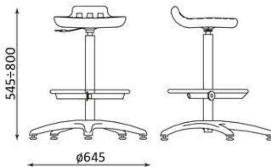
Taboret WORKER ring base - wymiary
